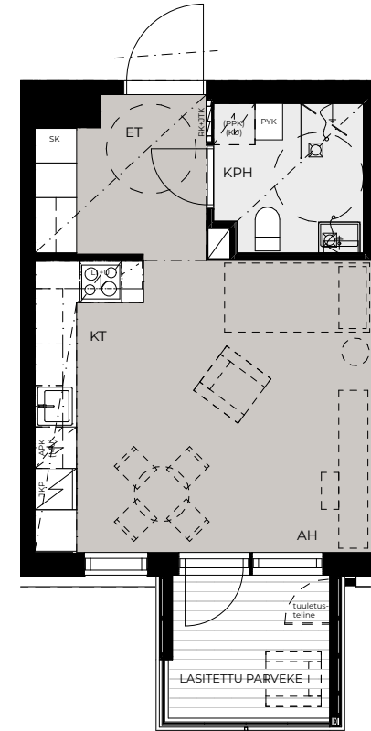
Pohjapiirustus 1:100
